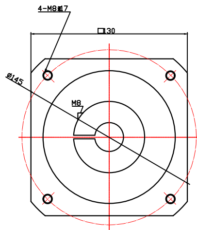
输入端
