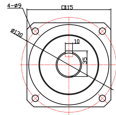
输出端
