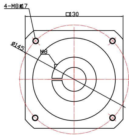
输入端
